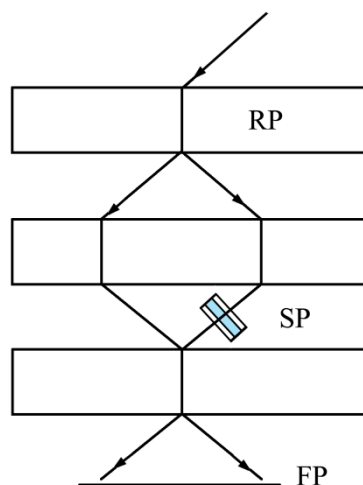
Рис.3. Ход лучей в LLL-интерферометре: RP – отражающие плоскости блоков, SP – исследуемый образец, FP – фотографическая пленка
